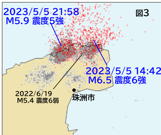
図3:震央分布図(2020年12月1日~2023年5月6日 M \geq 1.5) 赤丸:2023年5月5日~2023年5月6日に発生した地震 灰丸:赤丸以前に発生した地震
