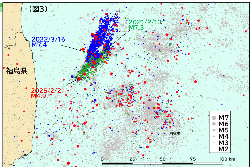
図3:震央分布図 (M \geq 2.0)
